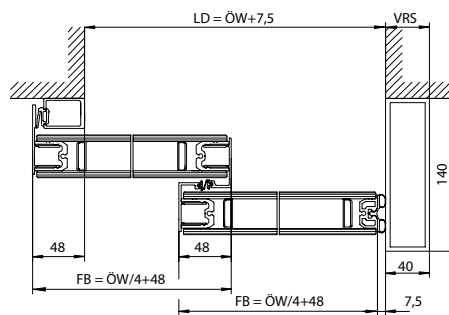
Вариант со створкой и боковыми частями DH = Высота прохода
