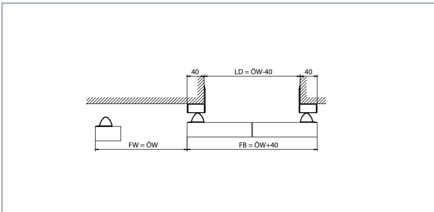
1-створчатая дверная система
