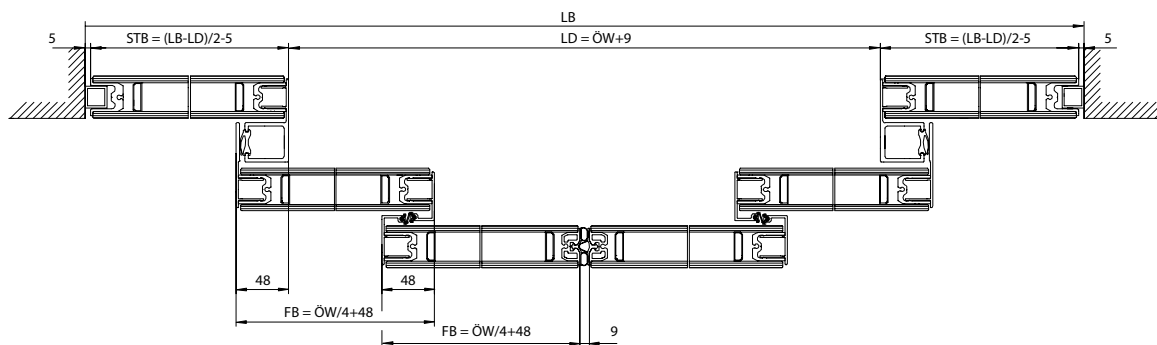
4-створчатая система дверей
