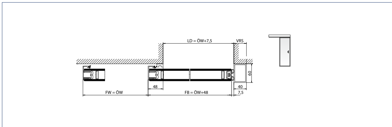
Напольная направляющая: Для монтажа в пол DH = Высота прохода
