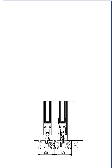
Напольная направляющая: непрерывная
