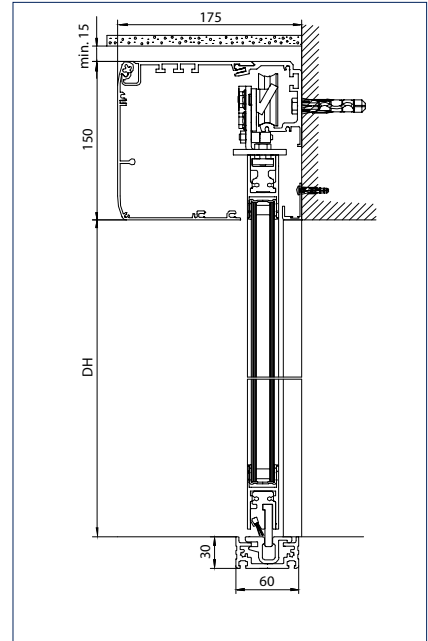
Напольная направляющая: непрерывная DH = Высота прохода
