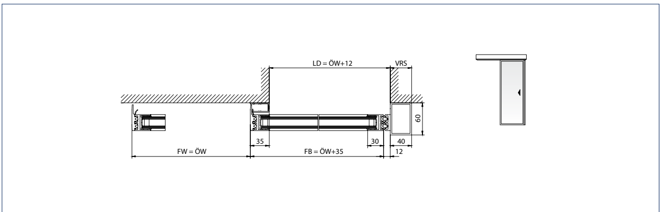
1-створчатая дверная система
